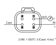
Deutsch DT04-4P
