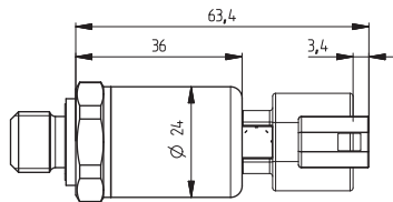
Deutsch DT04-3P
