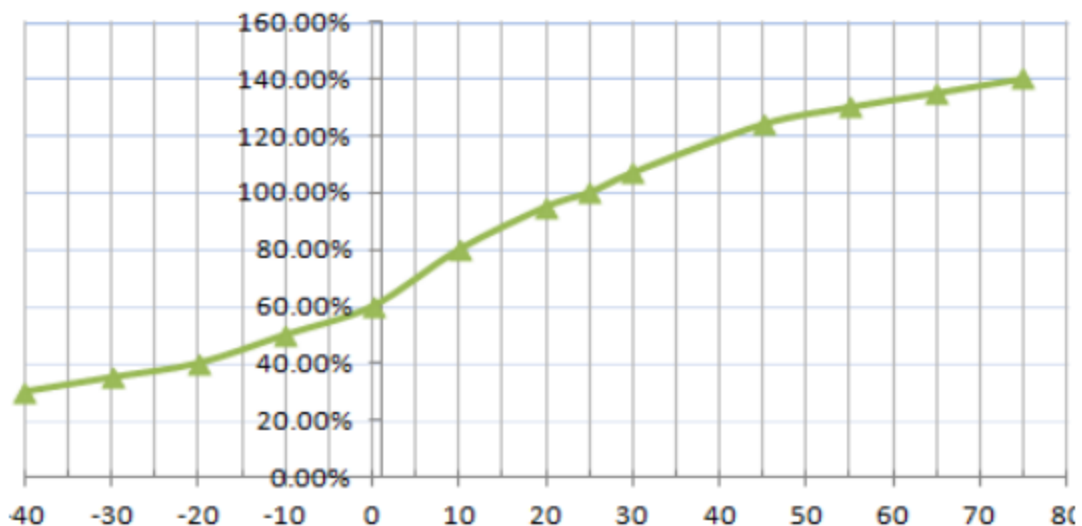
CO温度-灵敏度曲线
