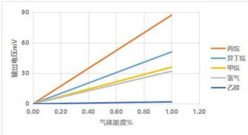
图 2 可燃气体灵敏度特性
