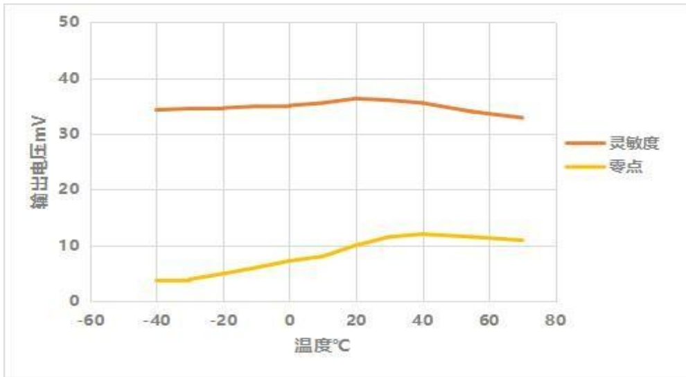
图 5 温度对零点、灵敏度的影响
