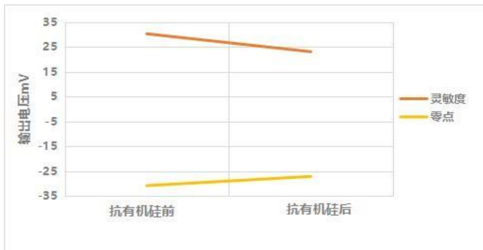
图 6 抗有机硅蒸汽能力
