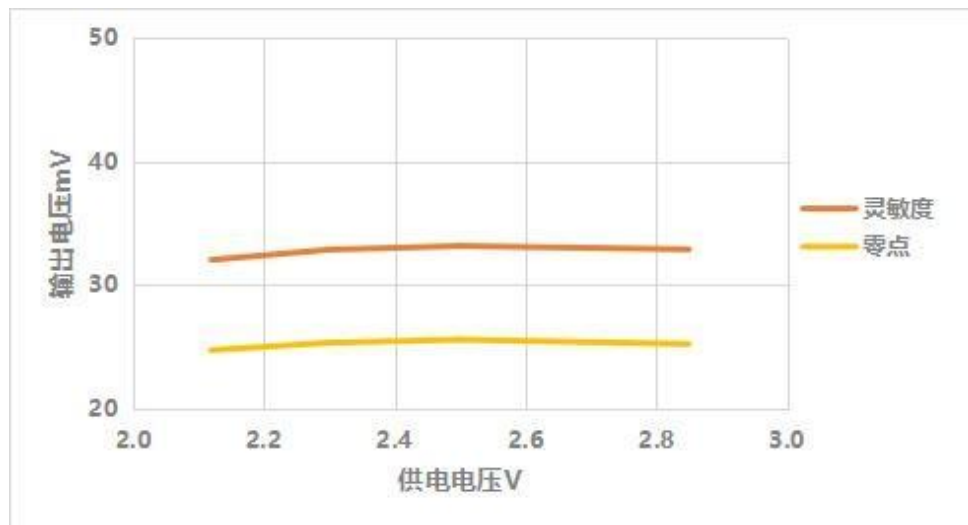
图 4 电压波动对零点、灵敏度的影响
