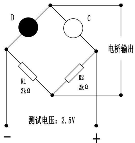
图 8 基本测试电路
