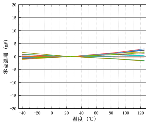
图 6 比例模式下零点温漂
