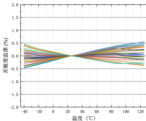
图 7 灵敏度温漂
