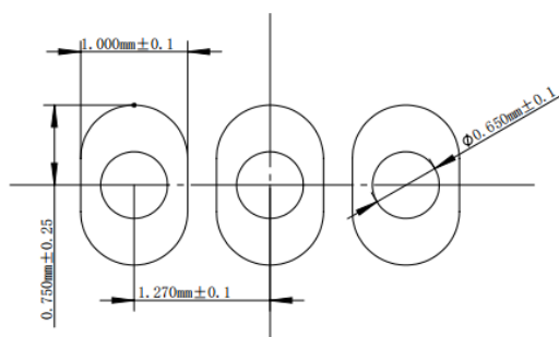
图 20 推荐焊盘尺寸
