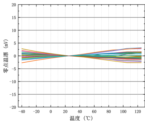
图 5 固定模式下零点温漂
