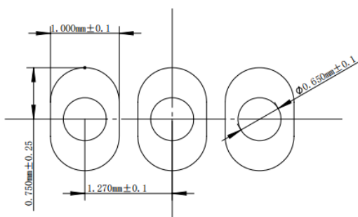
图 24 推荐焊盘尺寸
