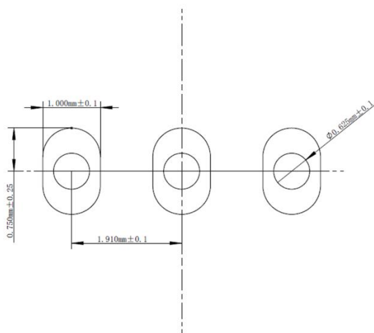
图 22 推荐焊盘尺寸
