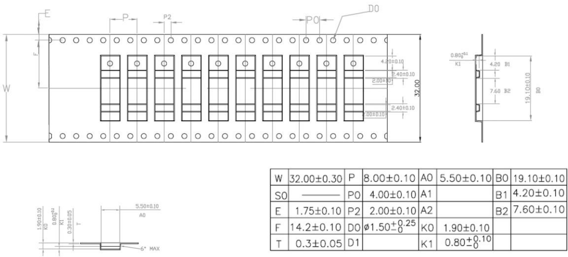
图 26 编带示意图
