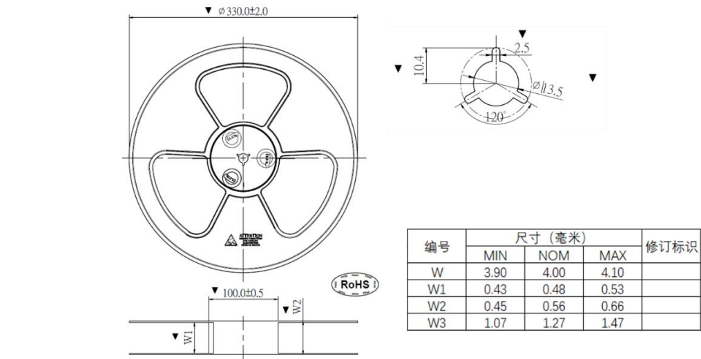
图 25 卷盘图
