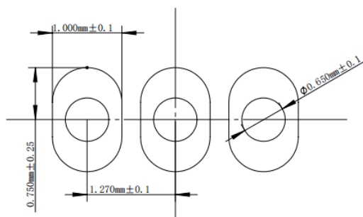
图 16 推荐焊盘尺寸
