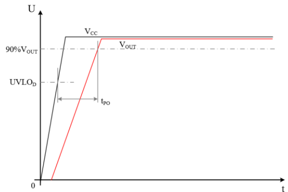
图 14 上电启动时间示意图
