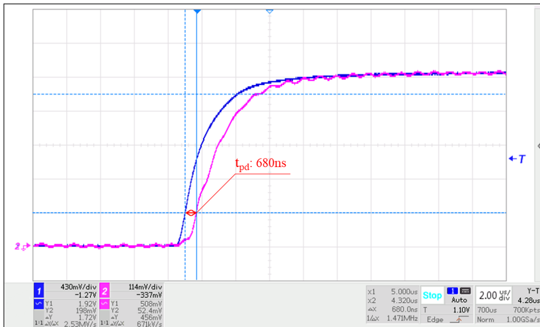
图 10 传输延迟时间测试图
