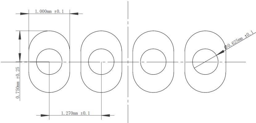
图 18 推荐焊盘尺寸
