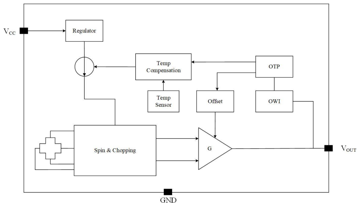
图 4 功能框图
