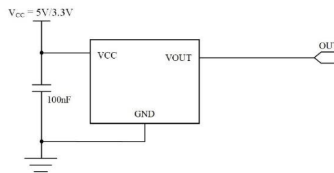
图 2 比例输出应用电路
