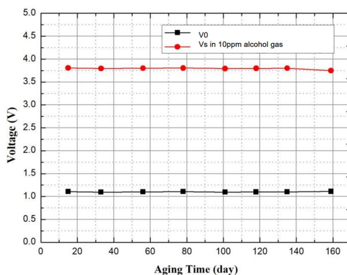
图 3 传感器的长期稳定性曲线
