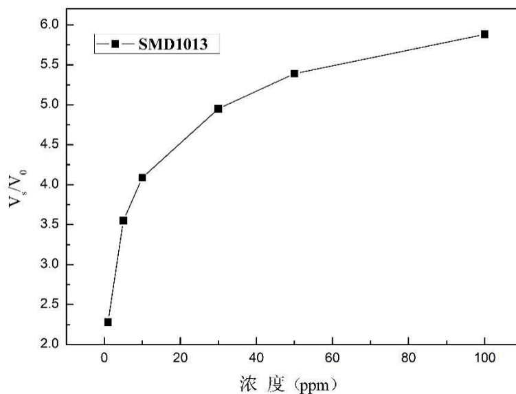
图1 传感器的灵敏度特性曲线
