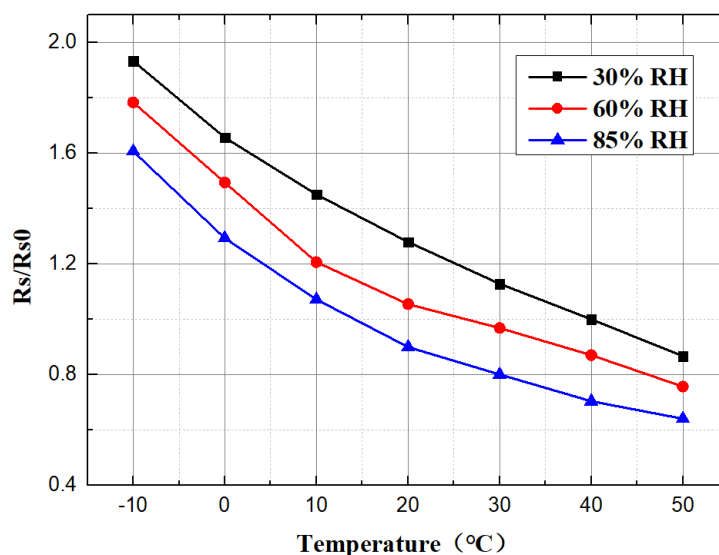
图2 传感器温度、湿度特性曲线
